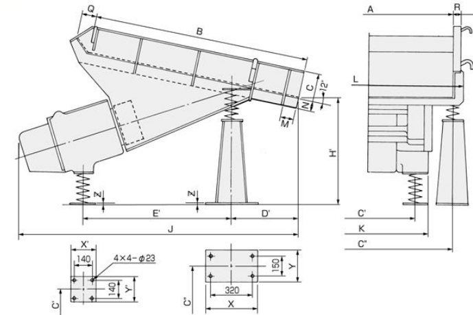
RFH-160B～1500B 下部駆動据置形
