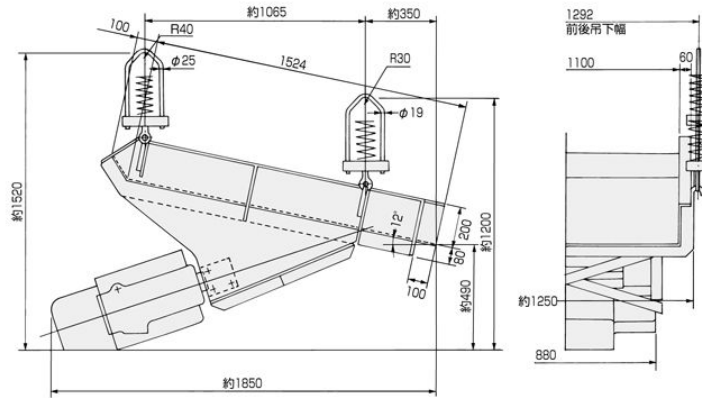
RFH-85B 下部駆動吊下形
