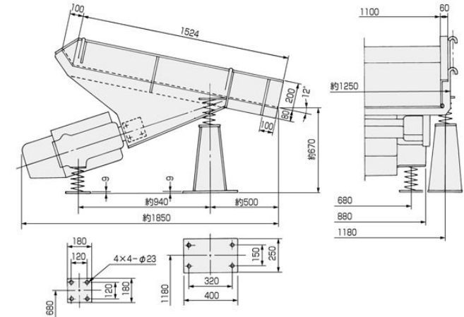
RFH-85B 下部駆動据置形
