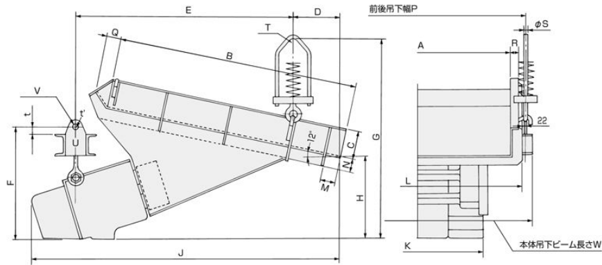
RFH-160B～1500B 下部駆動吊下形
